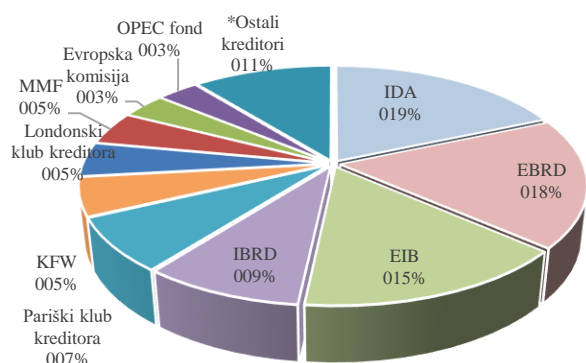
Grafikon 1. % učešća kreditora u servisiranim obavezama
